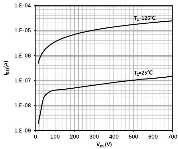
漏源级漏电流- V_{DS} 曲线
