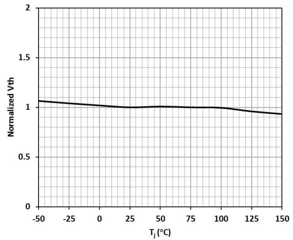
栅极阈值电压- T_j 曲线
