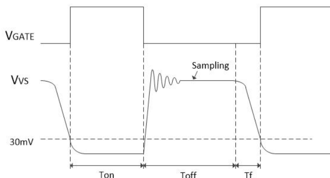
图 4 辅助绕组波形及退磁检测
