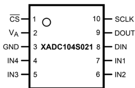
引脚图
