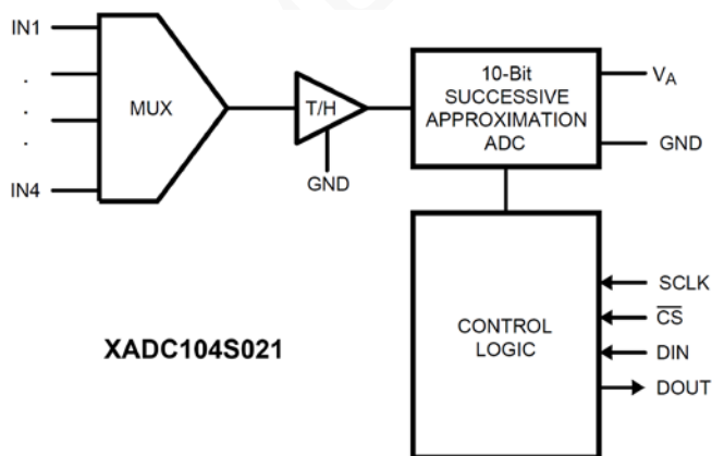
原理图
