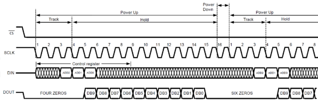
XADC104S021 操作时序图
