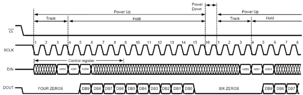
XADC108S022 操作时序图
