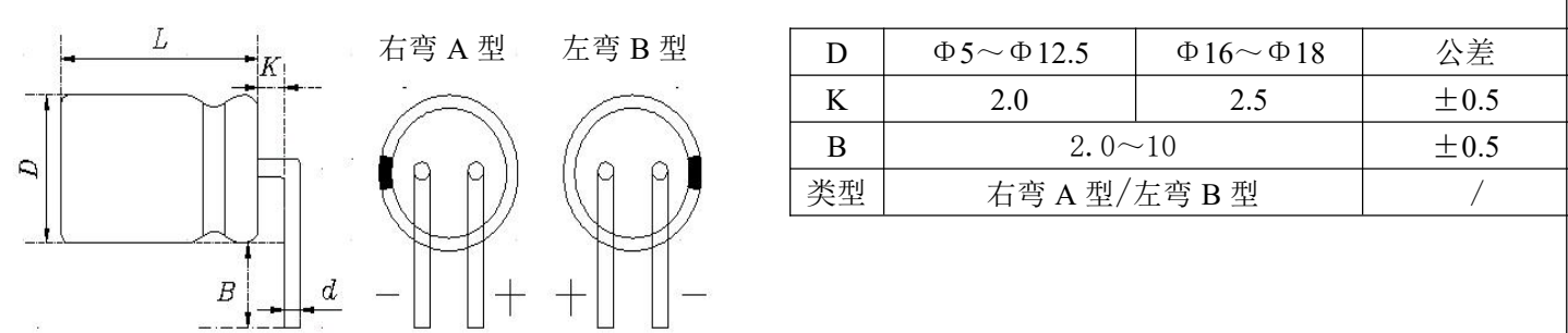
引线切脚成型 F 图（成型折弯 90°）
