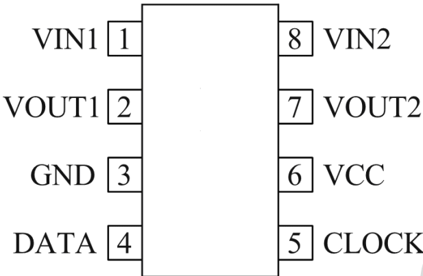
图 3、引脚排列
