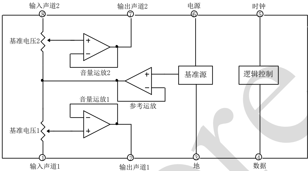
图 1、功能框图
