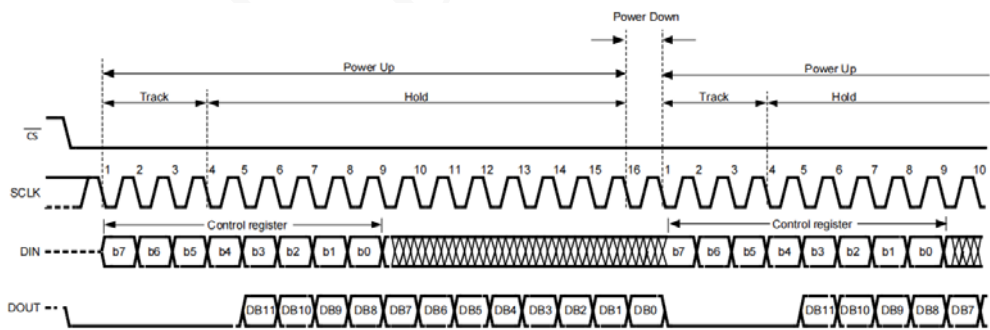
XADC122S051 操作时序图
