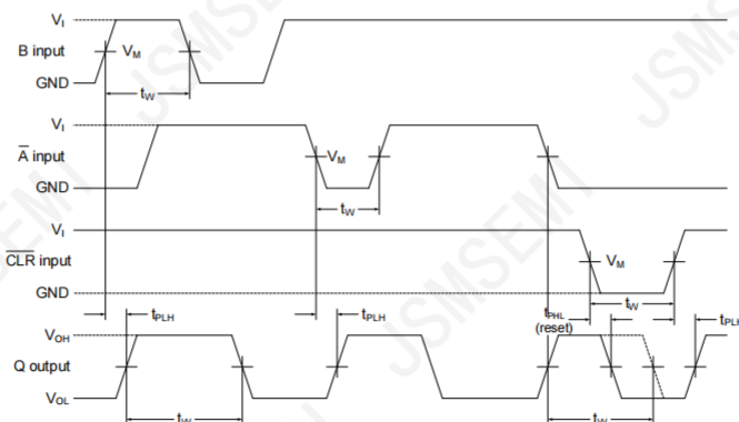
图4. 输入（ \overline{A} , B, \overline{CLR} ）到输出（Q）的传输延迟
