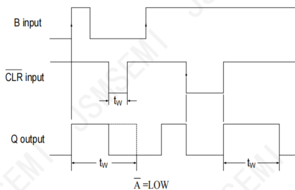
图6. 使用复位输入 \overline{\text{CLR}} 的脉宽控制
