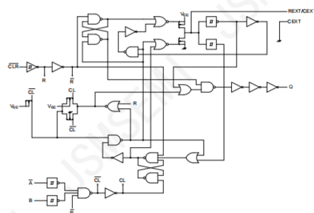
图 2. 逻辑示意图
