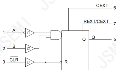
图 1. 逻辑符号
