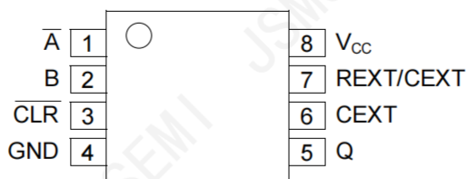
TSSOP8/VSSOP8
