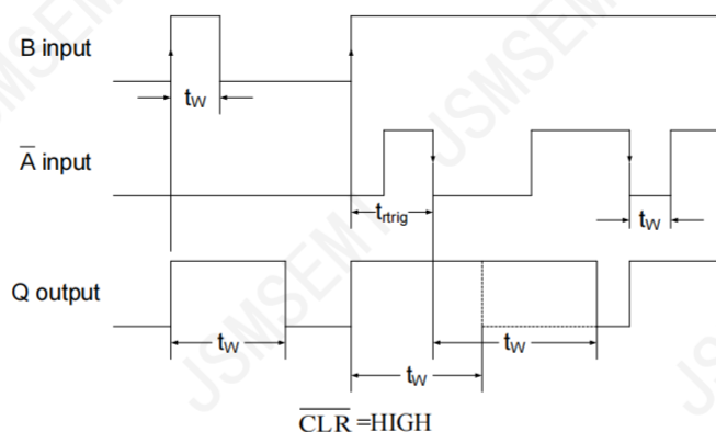
图5. 使用重复触发脉冲的脉宽控制
