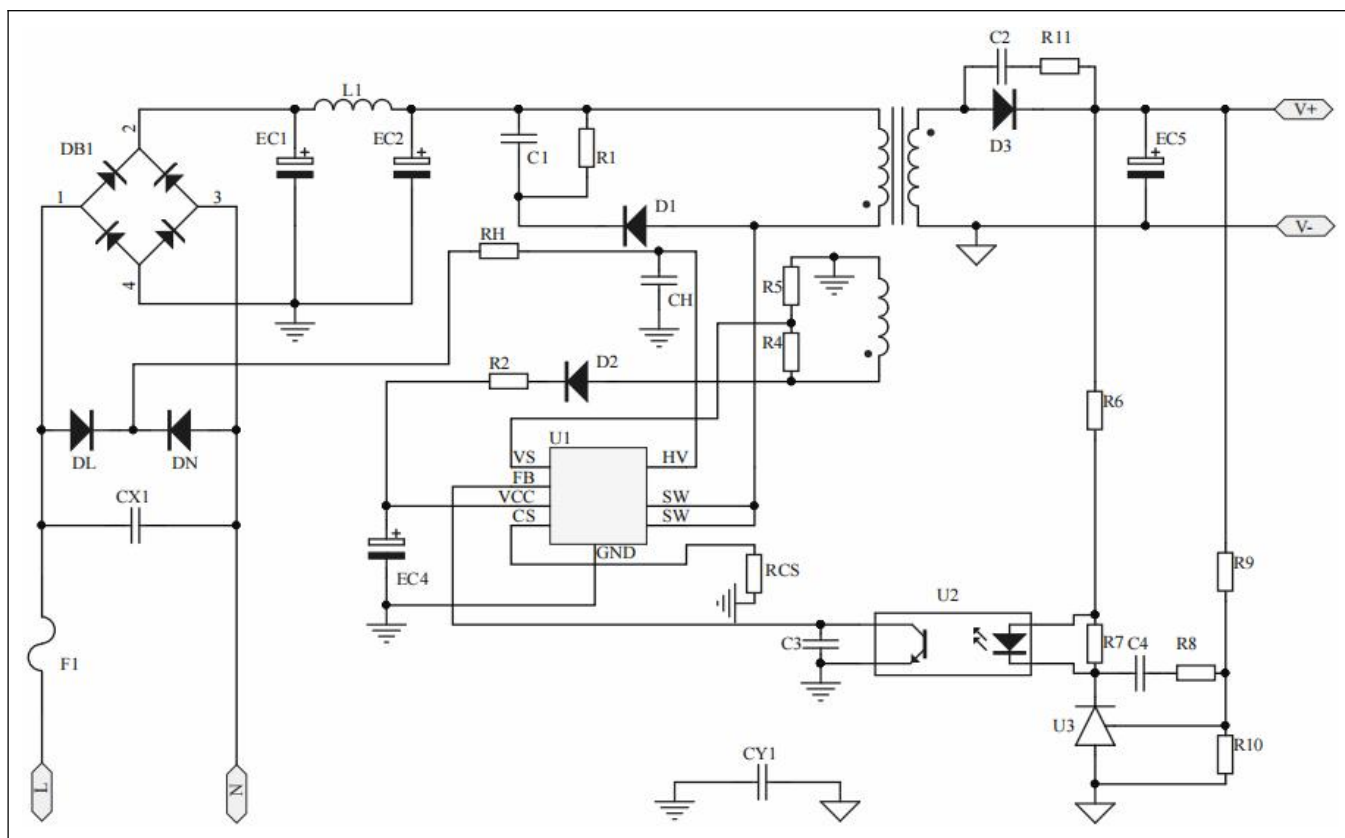
HV 带 X 电容放电功能电路图
