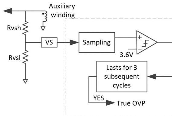
图 5 输出过压保护
