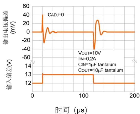
线性瞬态响应
