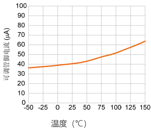
可调管脚电流 vs. 温度
