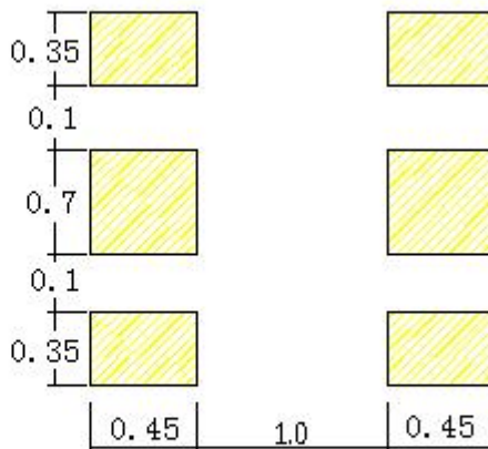
建议焊盘尺寸
