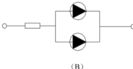
(B) 每个灯珠可能出现亮度不一致， 是由 I-V 的曲线而导致的。
