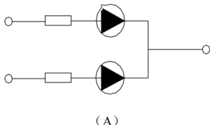
(A) 被推荐的电路
