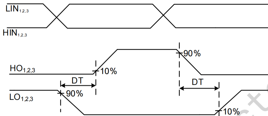
图 6-3 死区时间波形定义
