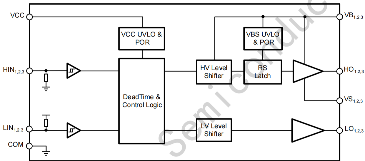
图 7-1 JSM6288功能框图
