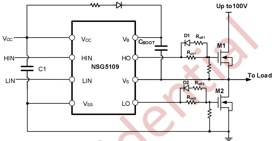
图 10-3 典型应用电路图
