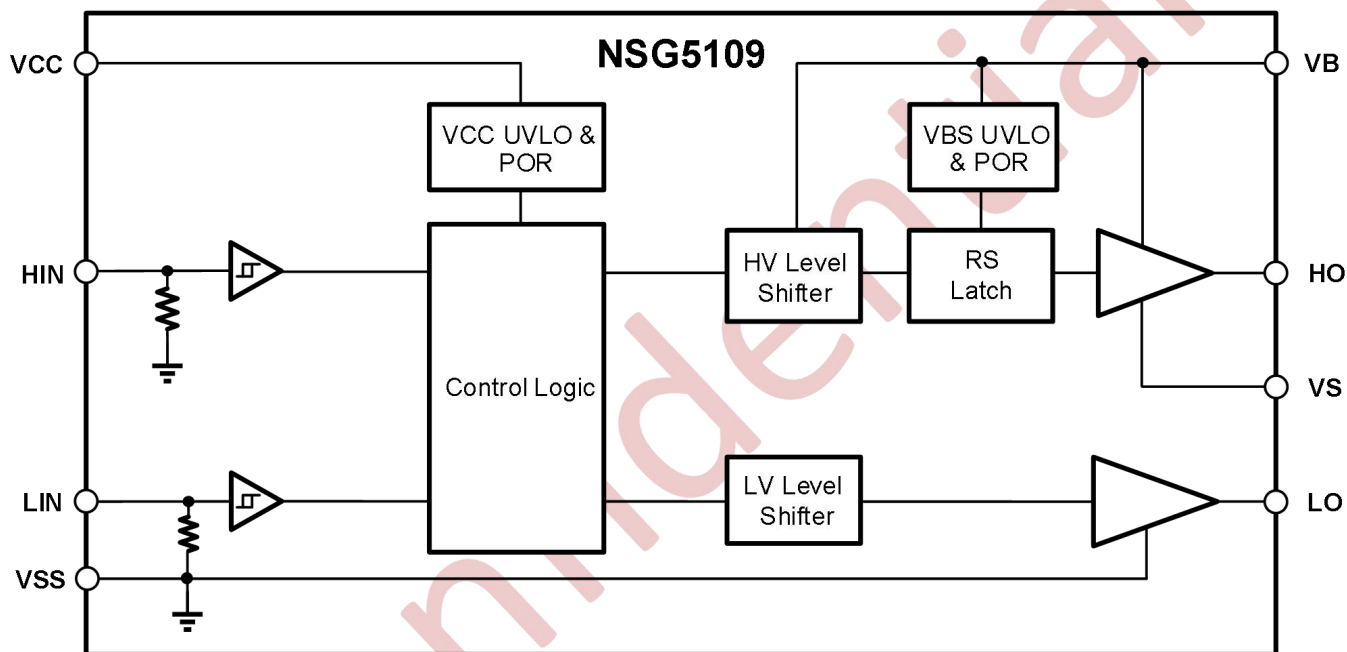
图 10-1 NSG5109 功能框图
