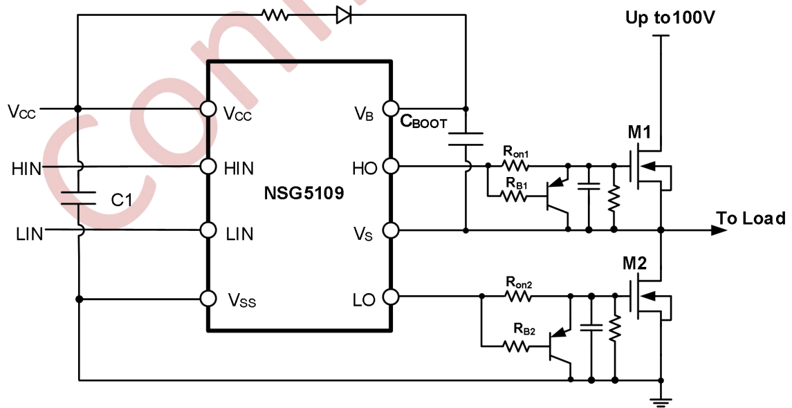
图 10-4 典型应用电路图
