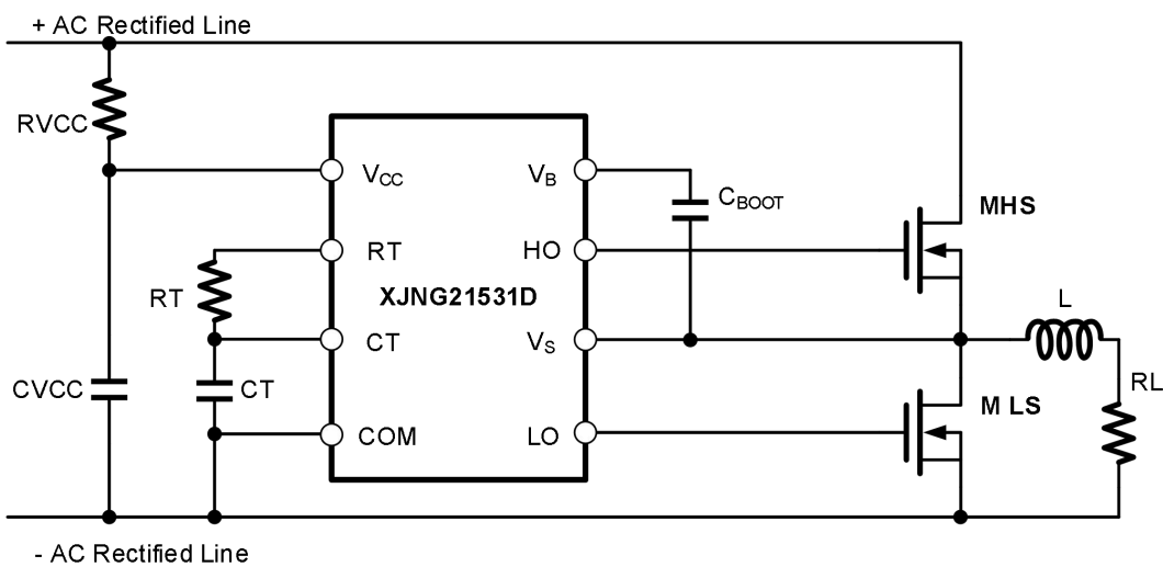
图 10-2 XJNG21531D 典型应用电路图
