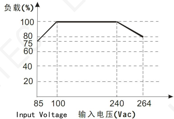
输入电压与负载关系图
