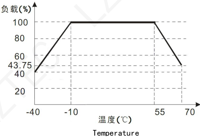
温度与负载关系图
