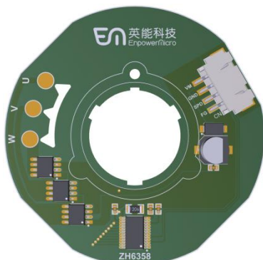
图 2 PCB 实景图
