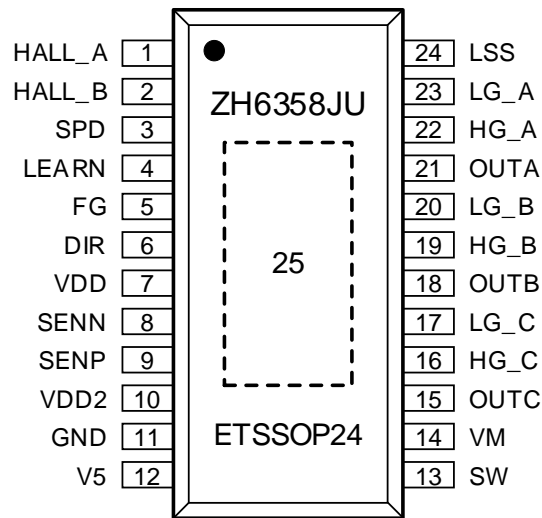
图 4 引脚分布
