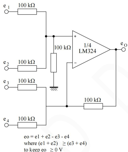
图 4：直流加法放大器
