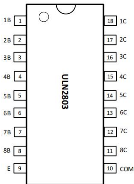
SOP18/DIP18 封装
