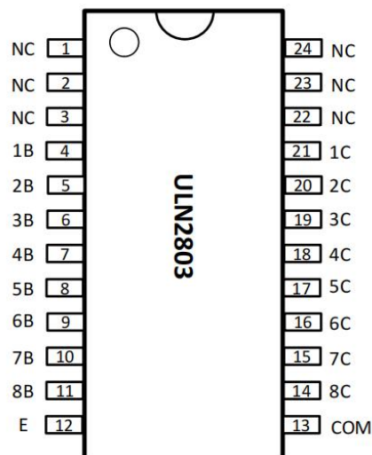
SSOP24 封装
