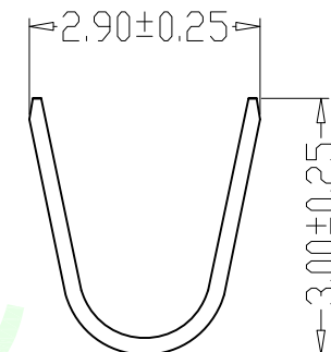
SEC:A-A
