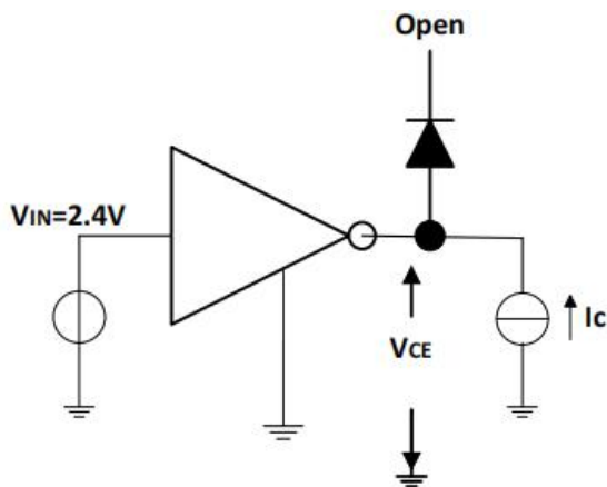
图 3 V_{CE(sat)} 测试电路
