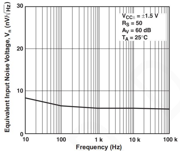
图 6 输入电压噪声与频率关系
