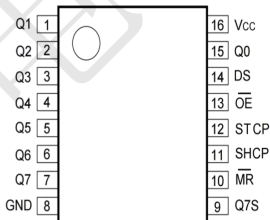
SOP-16
