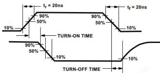
图 2 通道开启波形 ( R_L = 1\text{ k}\Omega )
