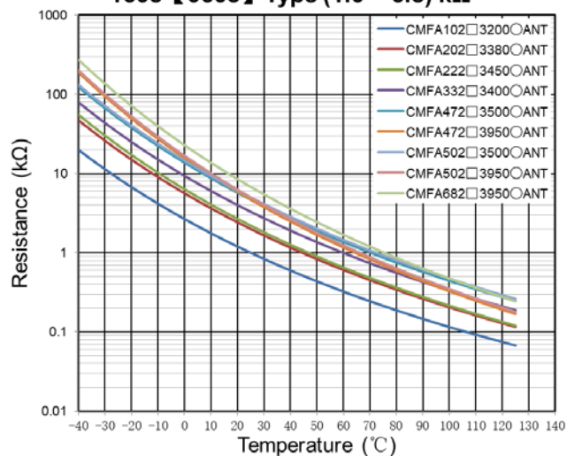
1608 【0603】 Type (1.0 ~ 6.8) kΩ
