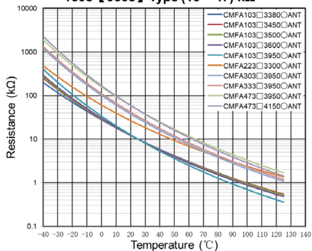
1608 【0603】 Type (10 ~ 47) kΩ
