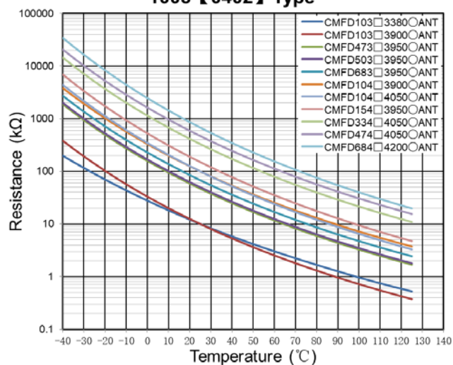
1005 【0402】 Type
