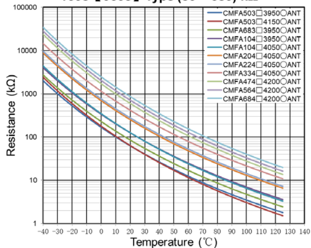
1608 【0603】 Type (50 ~ 680) kΩ
