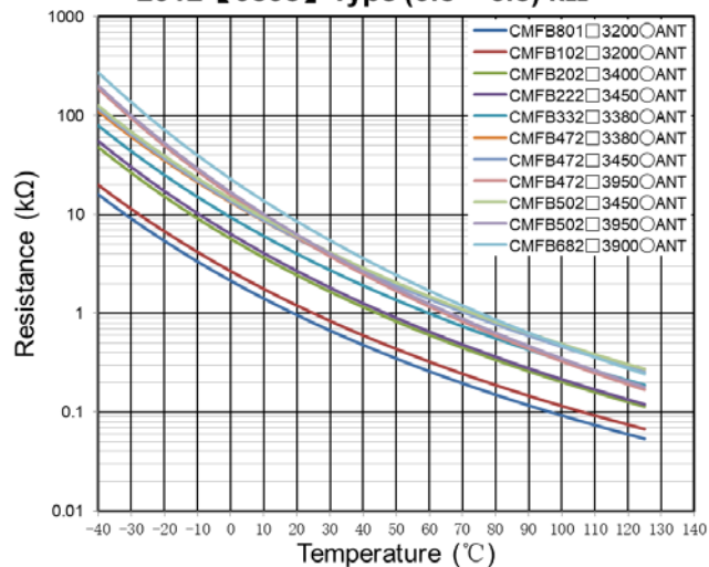
2012 【0805】 Type (0.8 ~ 6.8) kΩ
