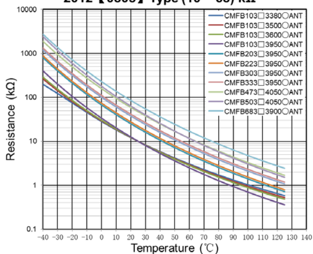
2012【0805】Type (10 ~ 68) kΩ
