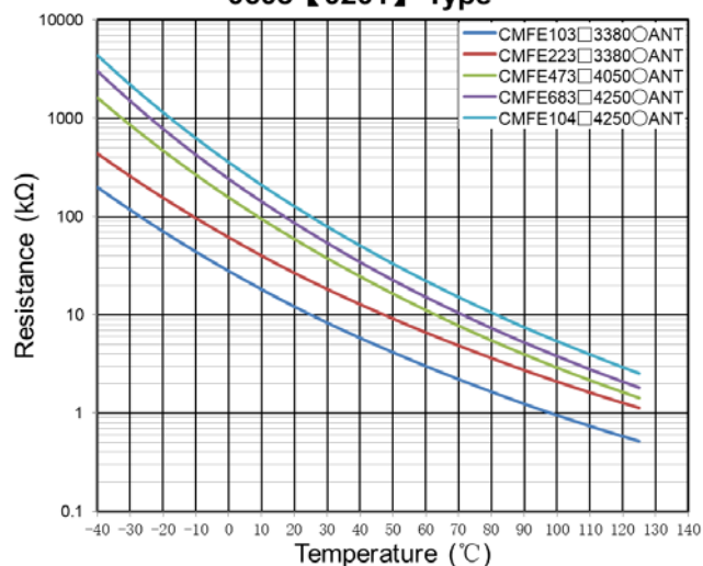
0603 【0201】 Type
