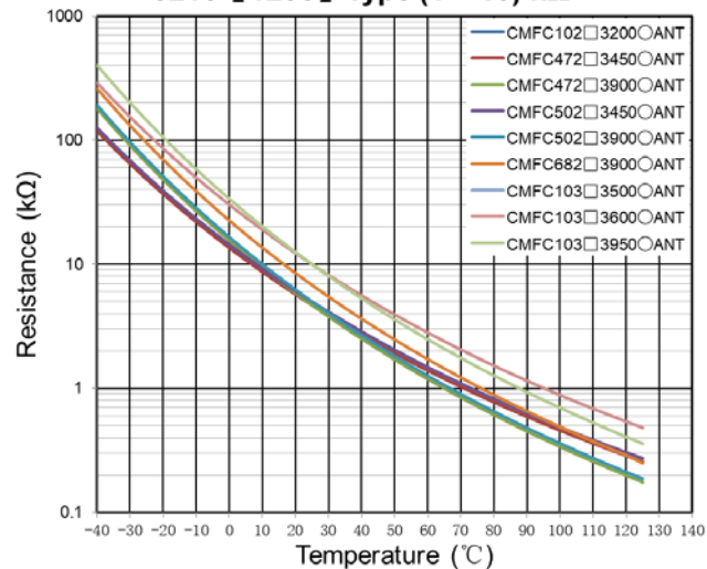
3216【1206】Type (1 ~ 10) kΩ
