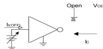
图 3 I(OFF) 测试电路图
