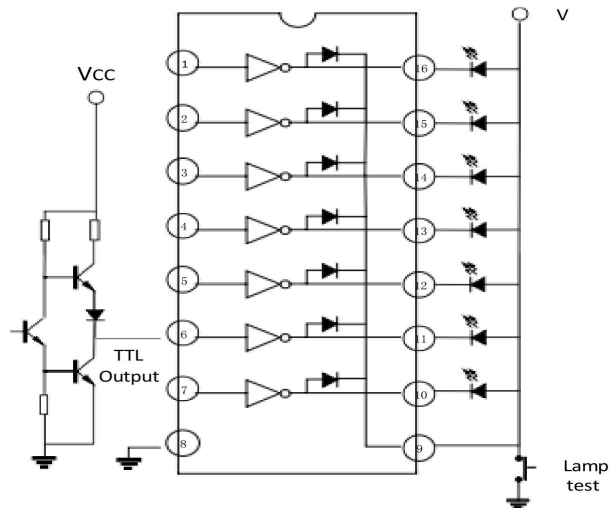
图 1 （ULN2003-TD）TTL 作为负载的应用电路图
