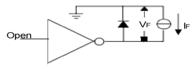
图 8 VF 测试电路图
