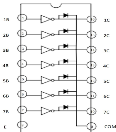
图 1 ULN2003-TD的逻辑框图
