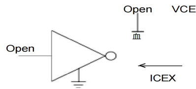
图 1 ICEX 测试电路图
