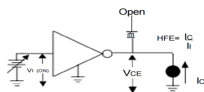
图 6 VI(ON)测试电路图
