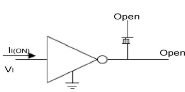
图 4 I(ON) 测试图
