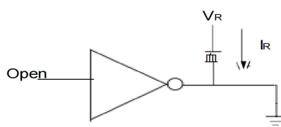
图 7 IR 测试电路图
