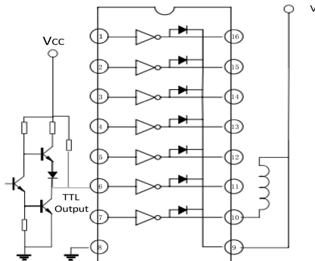
图 2 （ULN2003-TD）通过上拉电阻增加驱动电流的应用原理图
