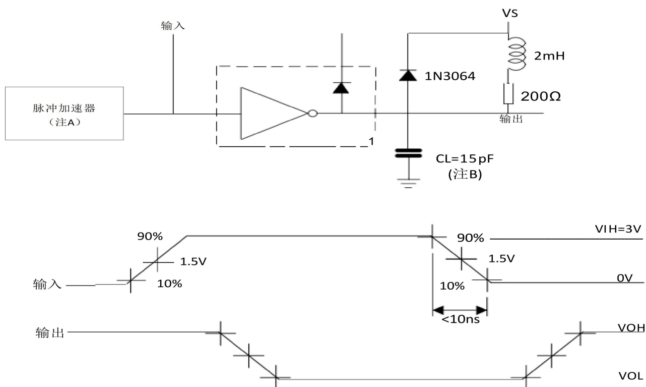
图 10 锁存测试电路图和电压波形
