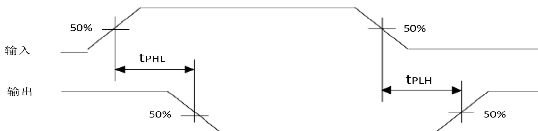
图 9 传播延迟时间波形
