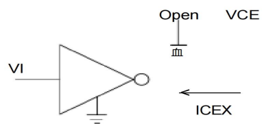
图 2 ICEX 测试电路图
