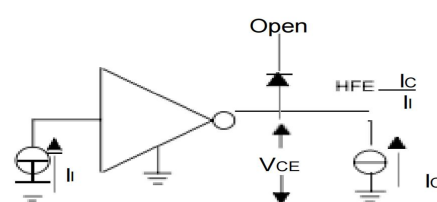
注：II是固定的测量VCE(SAT)，也可测量HFE 图 5 HFE, VCE(SAT) 测试电路图
