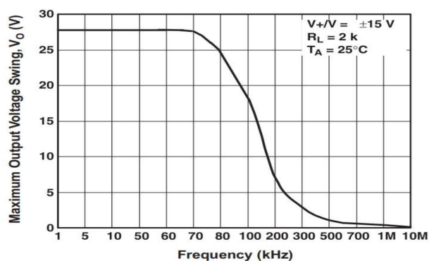
图 5 最大输出电压摆幅与频率关系
