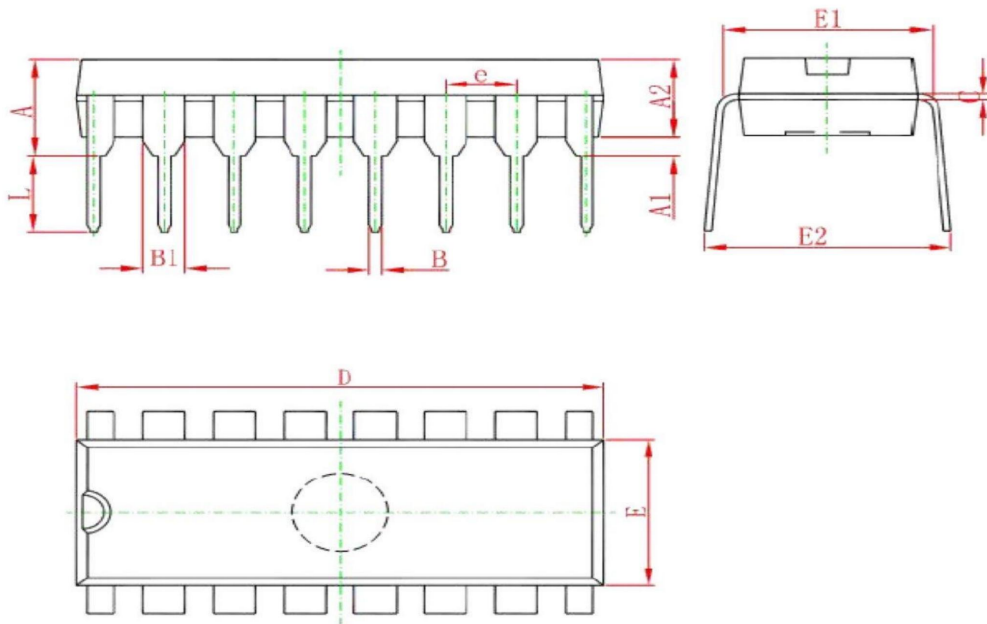
DIP16
