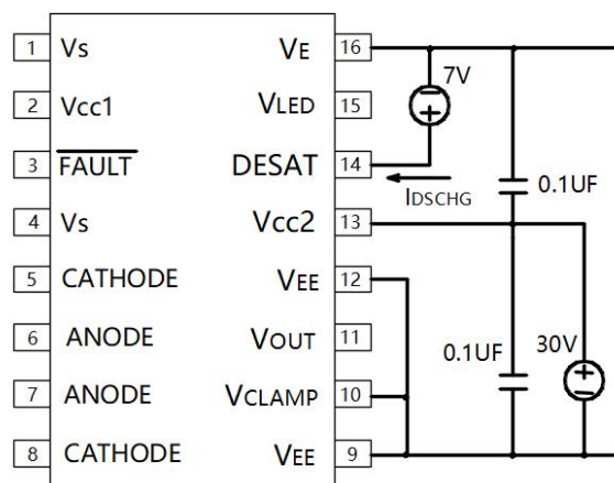
Fig28. IDSCHG Test Circuit
