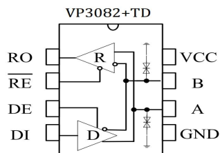
图 1 VP3082+TD引脚分布图
