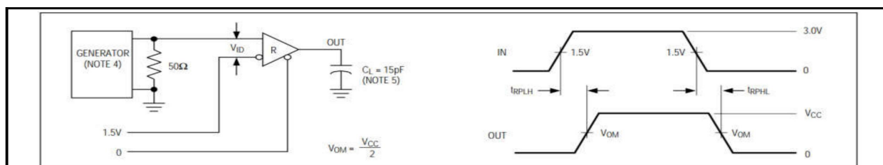
图 7 接收器传播延时测试电路
