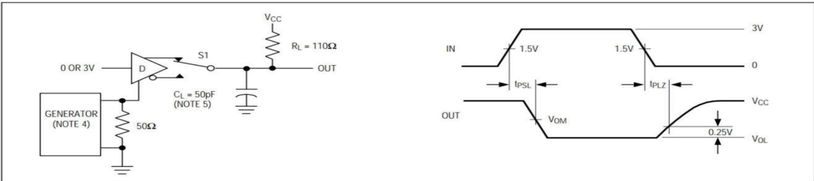
图 6 驱动器使能与禁能时间
