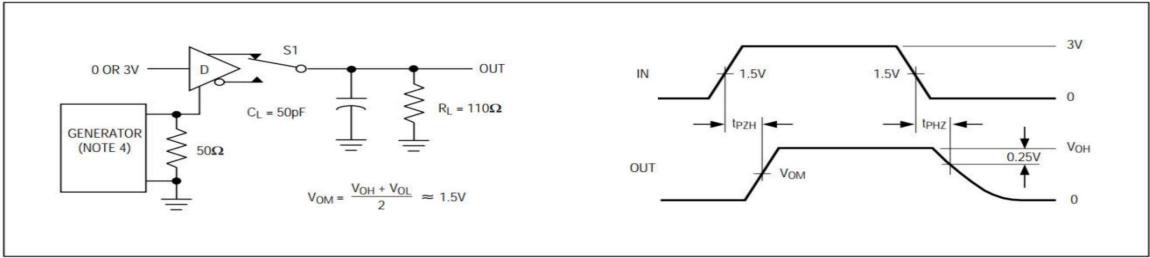
图 5 驱动器使能与禁能时间
