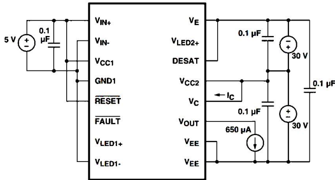
Fig49. ICH test circuit
