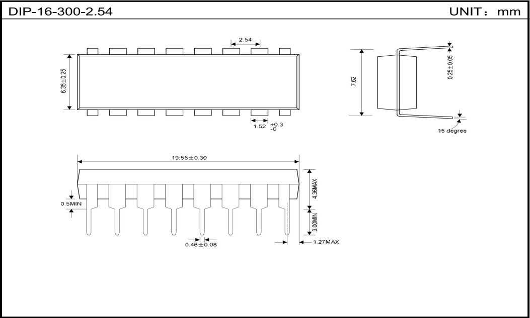
封装外形图
