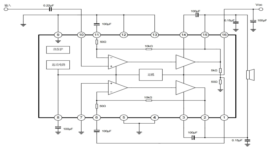
桥式应用电路
