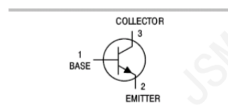
SOT-23
