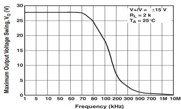
图 5 最大输出电压摆幅与频率关系
