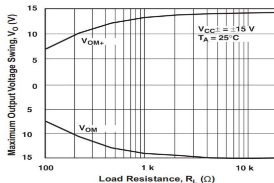
图 4 最大输出电压摆幅与负载关系
