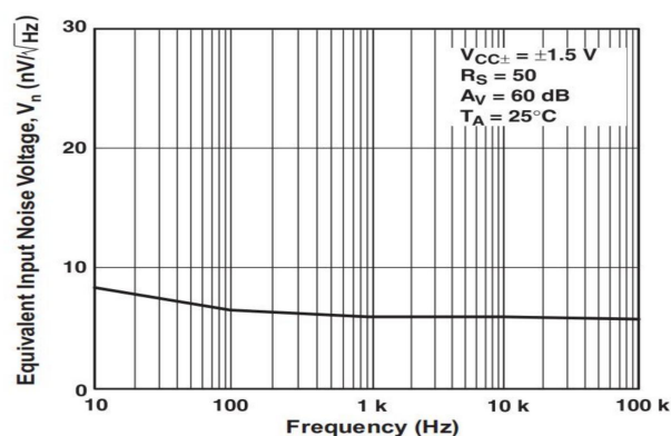
图 6 输入电压噪声与频率关系
