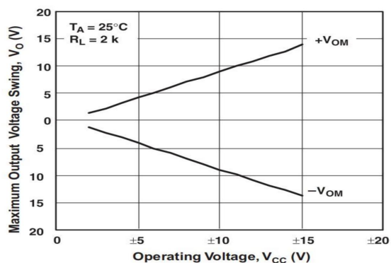
图 3 最大输出电压摆幅与电源电压关系
