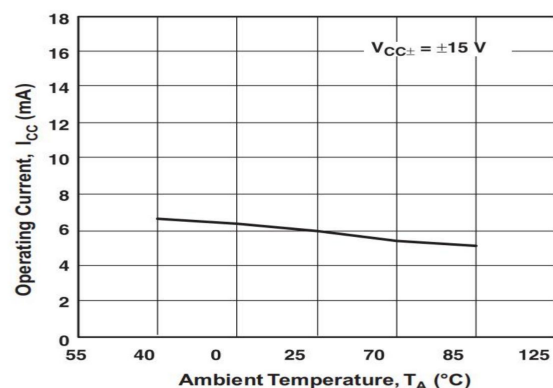
图 2 电源电流与环境温度关系
