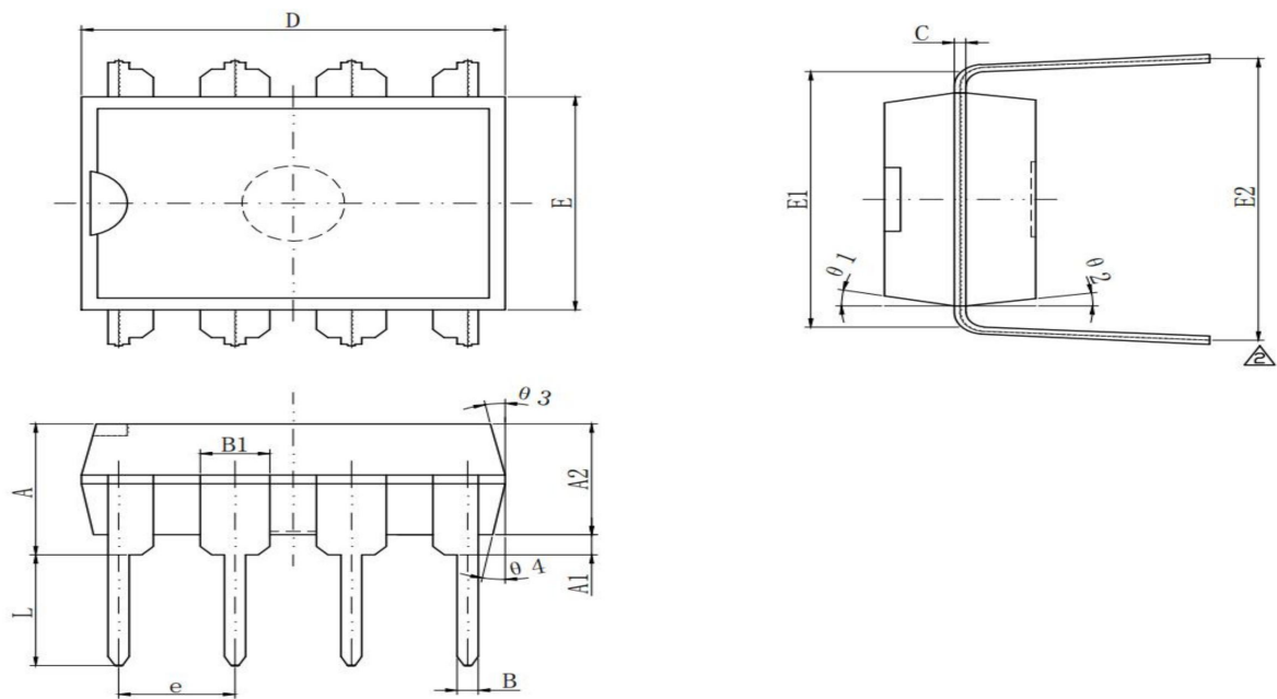
DIP8封装
