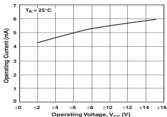
图 1 电源电流与电源电压关系
