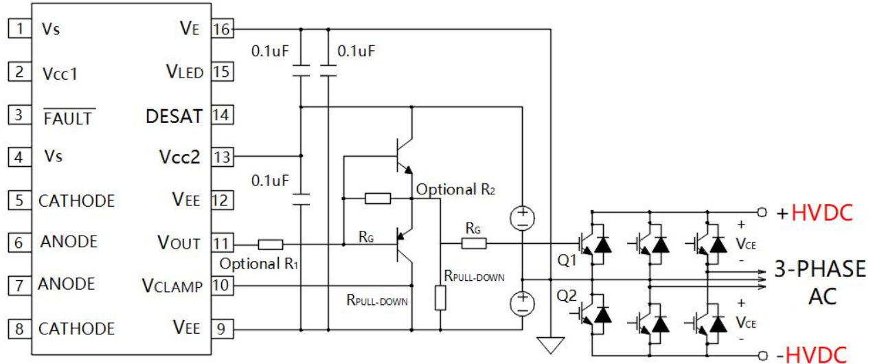
图.40 具有负栅极驱动，外部增压器的大型 IGBT 驱动。用于更高功率应用的 VCLAMP 控制二级放电路径
