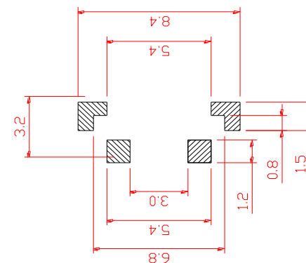
PCB. 焊接图
