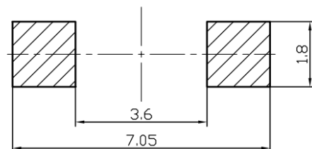
安装参考图
