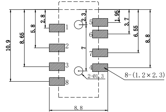
电路板开孔尺寸
