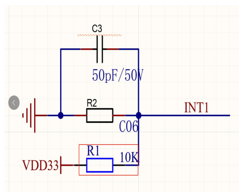
滤波电路
