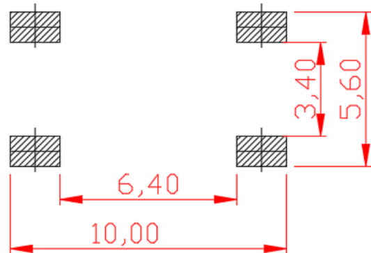
PCB. 焊接图
