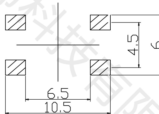
P.C.B焊接图G 供参考
