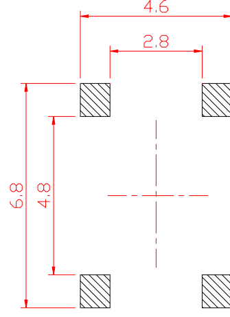
PCB. 焊接图
