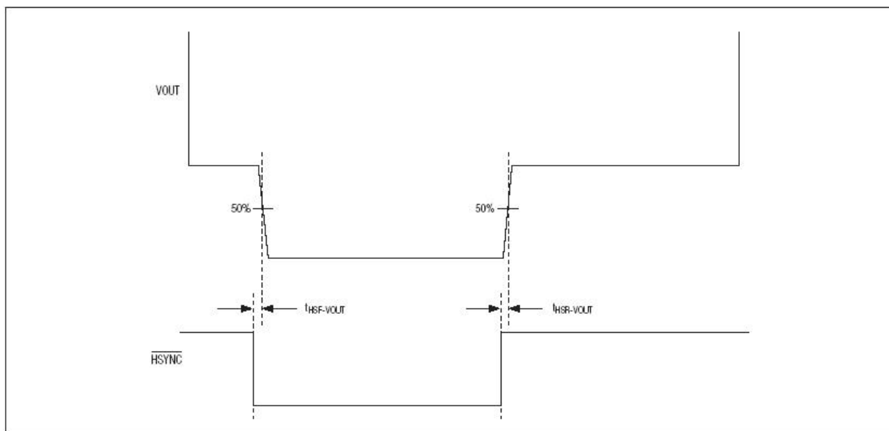
图9. VOUT和HSYNC行同步时序(NTSC和PAL, 内同步模式)
