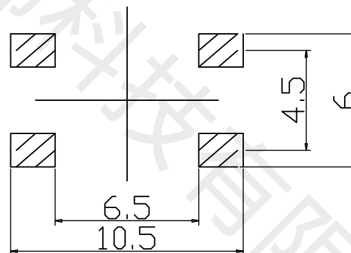
P.C.B焊接图 供参考
