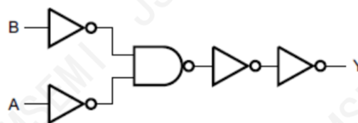
图 2 逻辑框图
