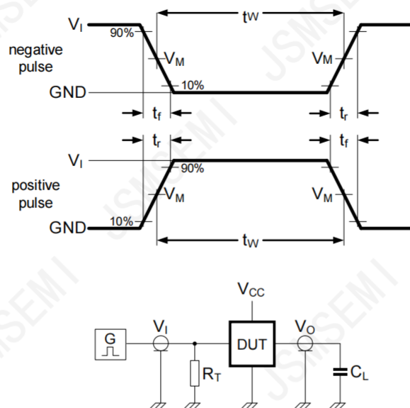
图4 测量开关时间的测试电路
