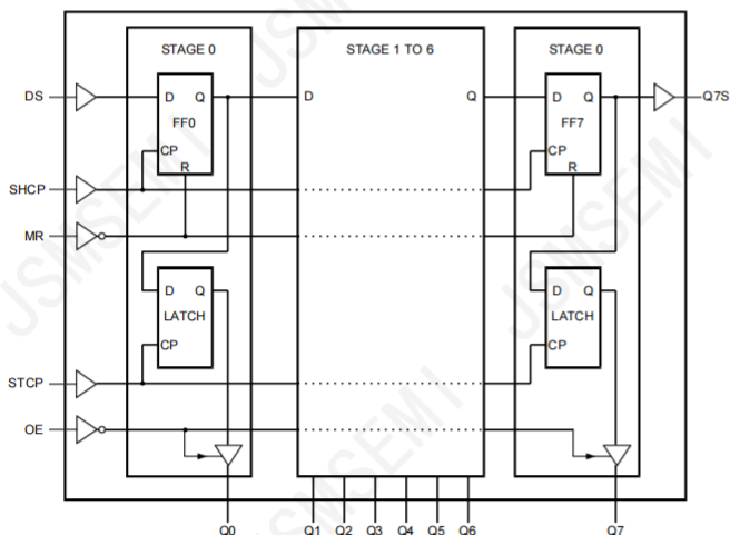
图 3 逻辑框图
