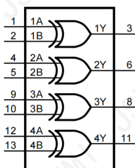
图1 逻辑符号
