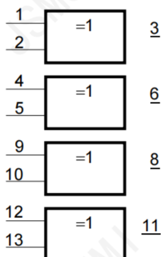
图2 IEC 逻辑符号
