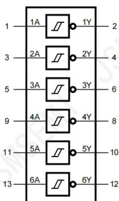
图 1 逻辑符号
