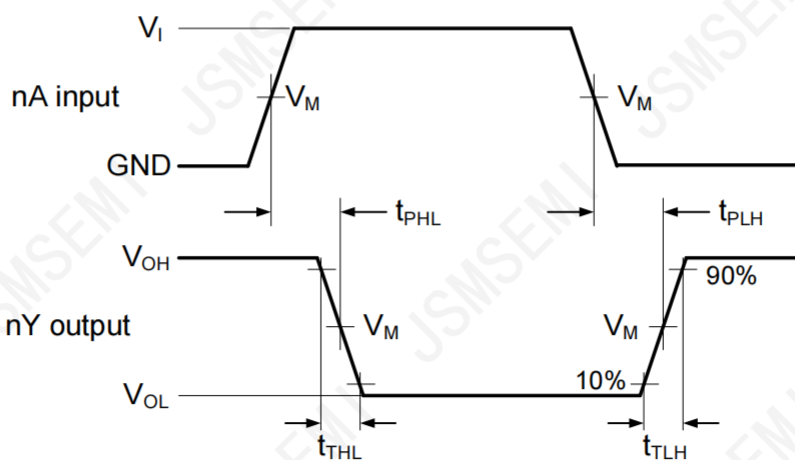
图5 输入到输出的传输延迟
