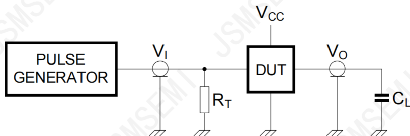
图4开关时间的负载电路
